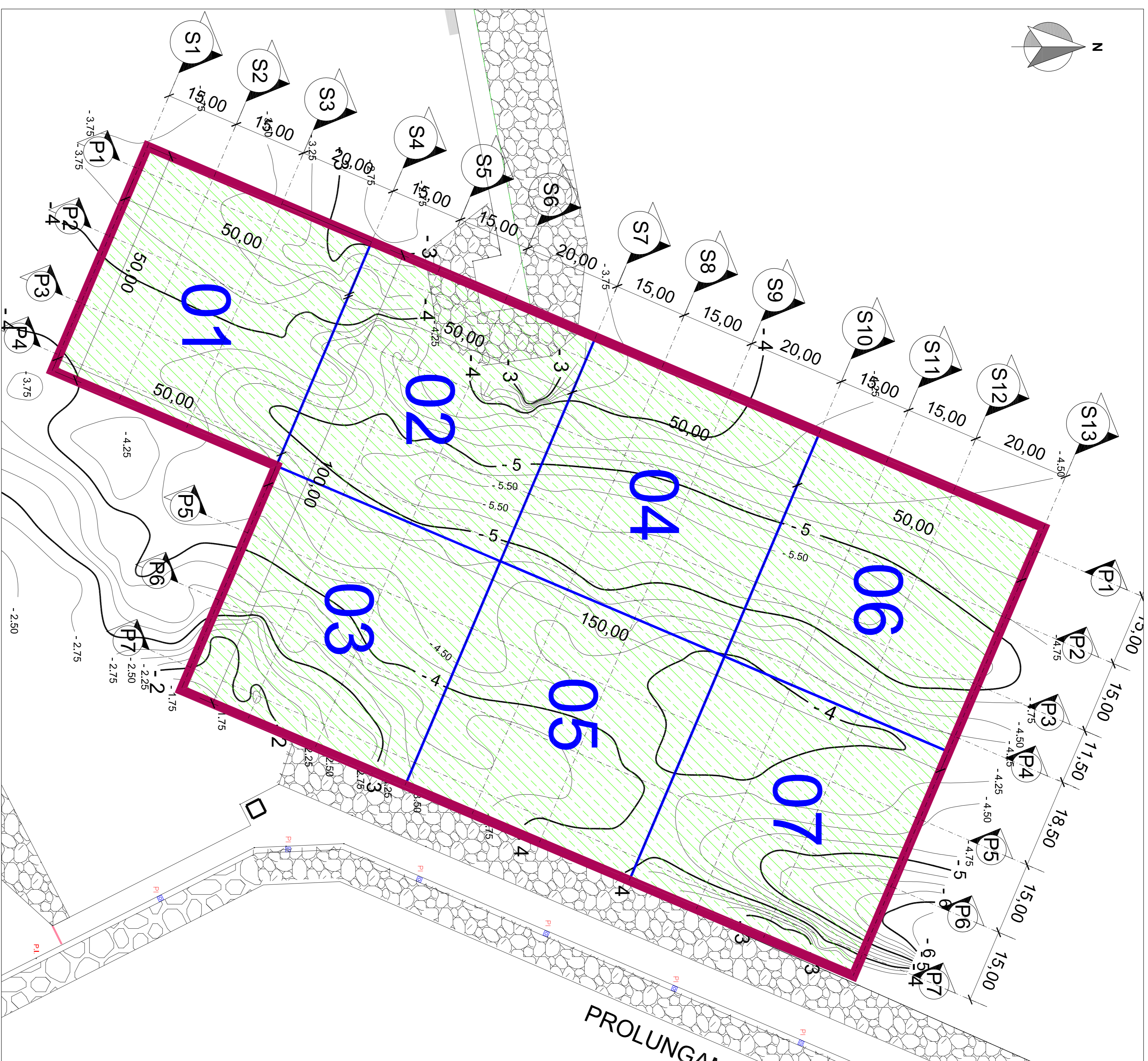
PLANIMETRIA CON BATTIMETRIE scala 1:500
